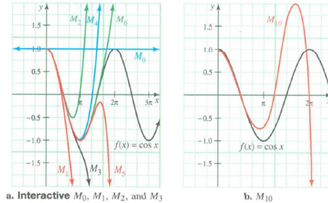
Hình 8.23. Hàm f(x) = \cos x và các đa thức Maclaurin của nó
