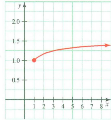
Hình 8.7. Đồ thị của hàm y = \sqrt{x^2 + 3x} - x, x \geq 1
